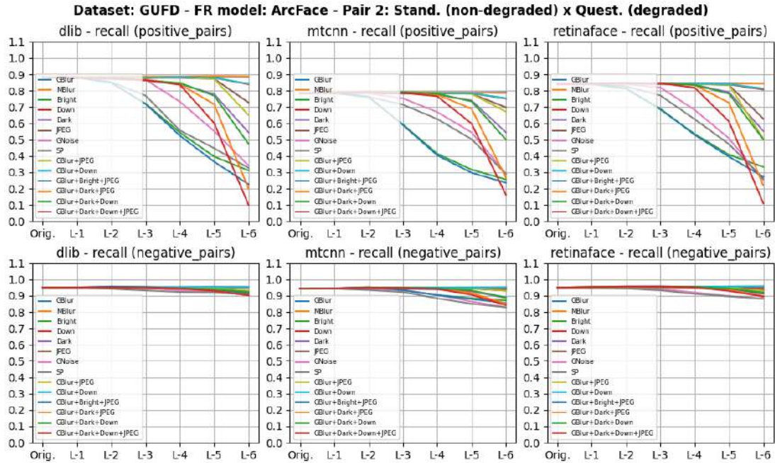
Figura I.57: Dataset GUFd - Par 2 - Métrica recall do algoritmo ArcFace
