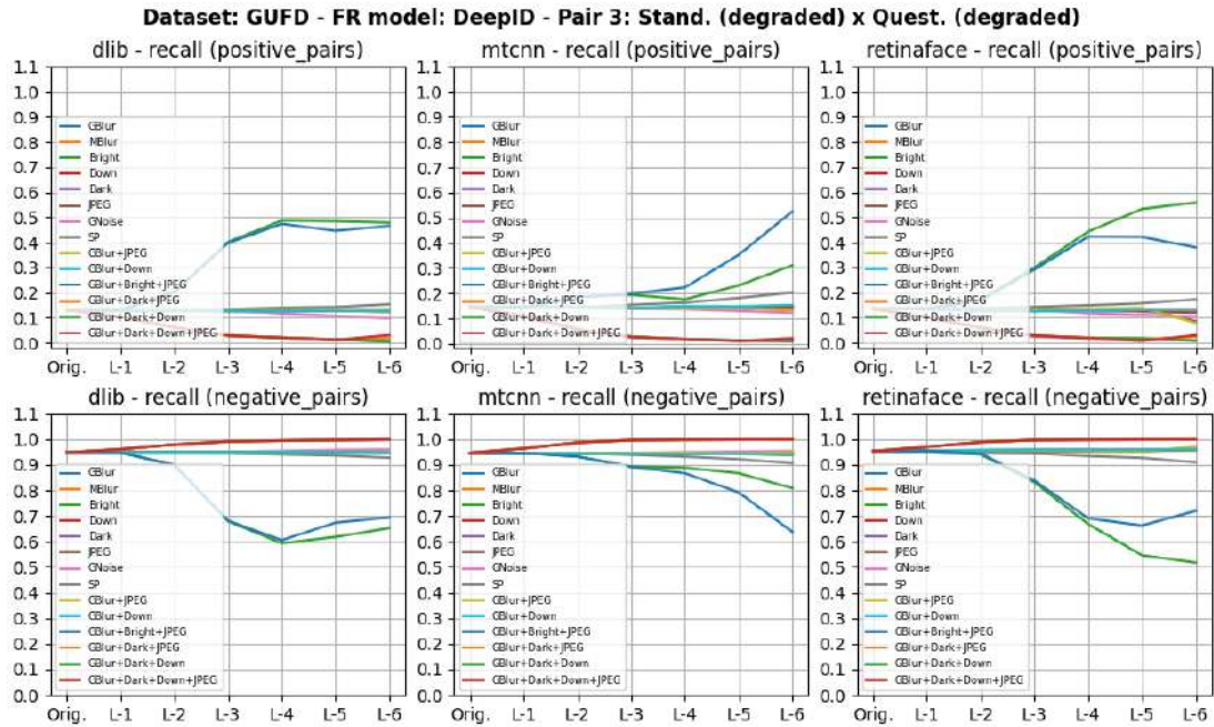
Figura I.67: Dataset GUFU - Par 3 - Métrica recall do algoritmo DeepID
