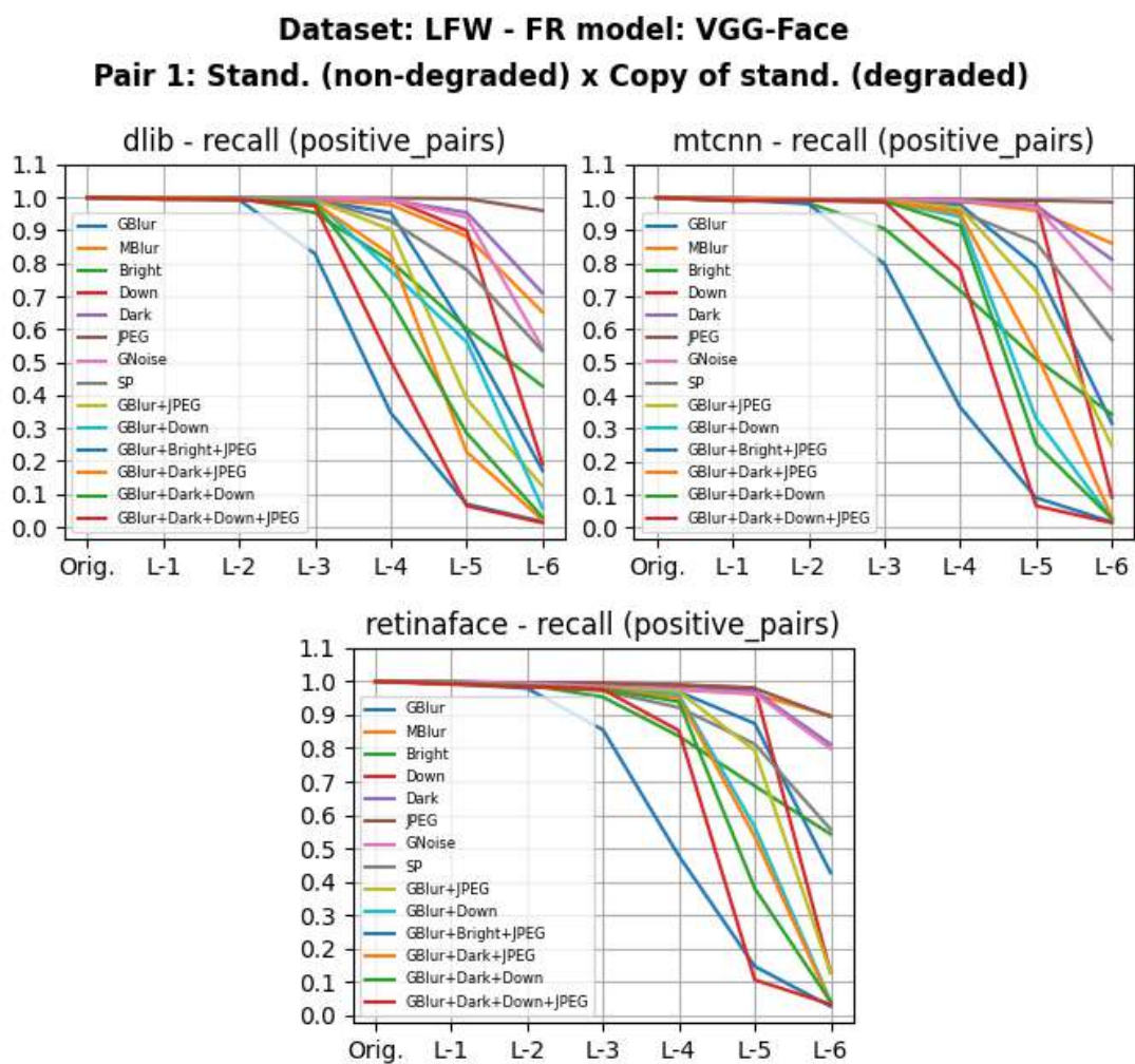
Figura 5.1: Métrica revocação do algoritmo VGG.
