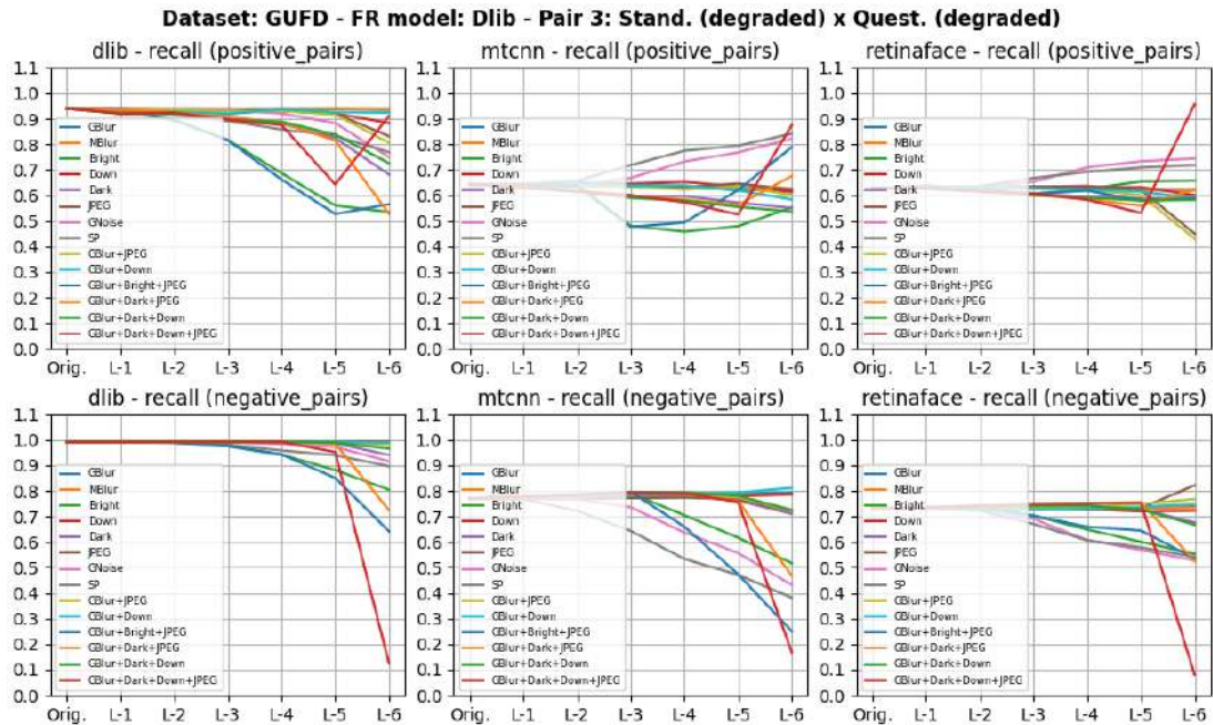
Figura I.68: Dataset GUFU - Par 3 - Métrica recall do algoritmo Dlib
