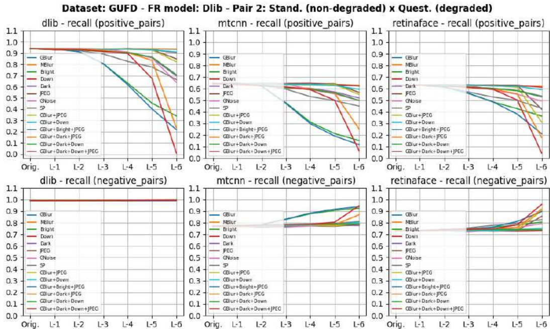
Figura I.60: Dataset GUF - Par 2 - Métrica recall do algoritmo Dlib
