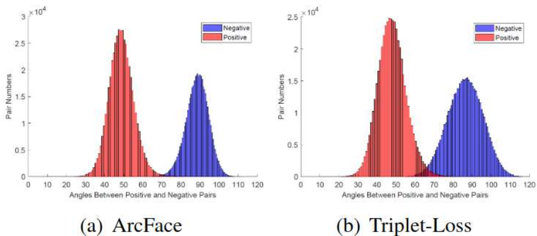
Figura 2.18: Distribuição das funções ArcFace e Triplet-loss. (Imagem extraída de [17])
