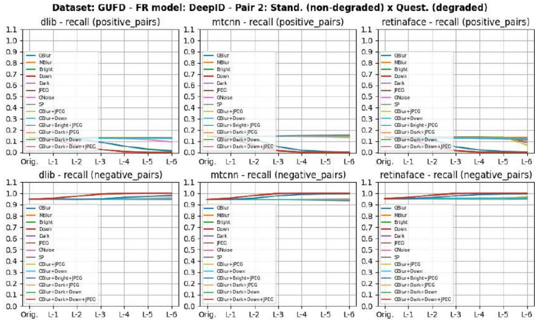
Figura I.59: Dataset GUF - Par 2 - Métrica recall do algoritmo DeepID
