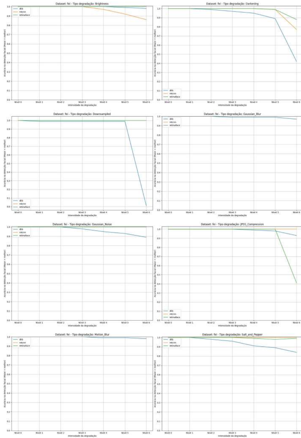
Figura I.99: Desempenho dos algoritmos de detecção facial (degradações simples) no dataset FEI
