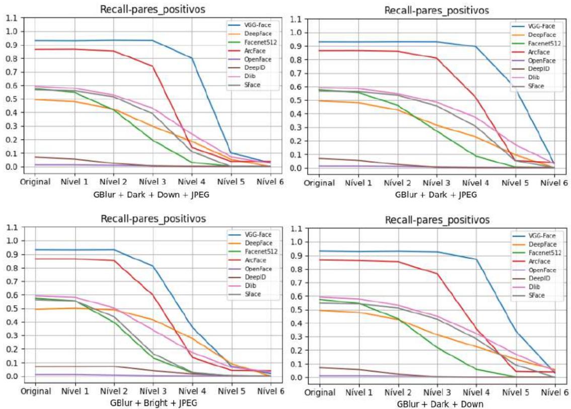
Figura 5.7: Maiores impactos para o Par 2 (todos os modelos) (mtcnn).
