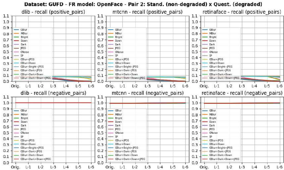
Figura I.62: Dataset GUF - Par 2 - Métrica recall do algoritmo OpenFace
