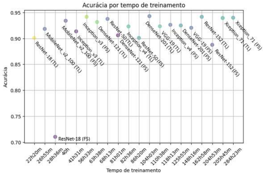
Figura 5.13: Acurácia x Tempo de treinamento para 100 épocas.
