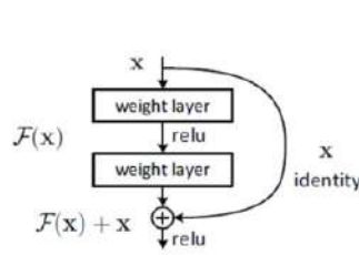
(d) ResNet
