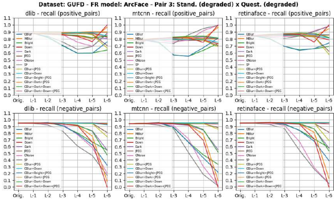
Figura I.65: Dataset GUFU - Par 3 - Métrica recall do algoritmo ArcFace
