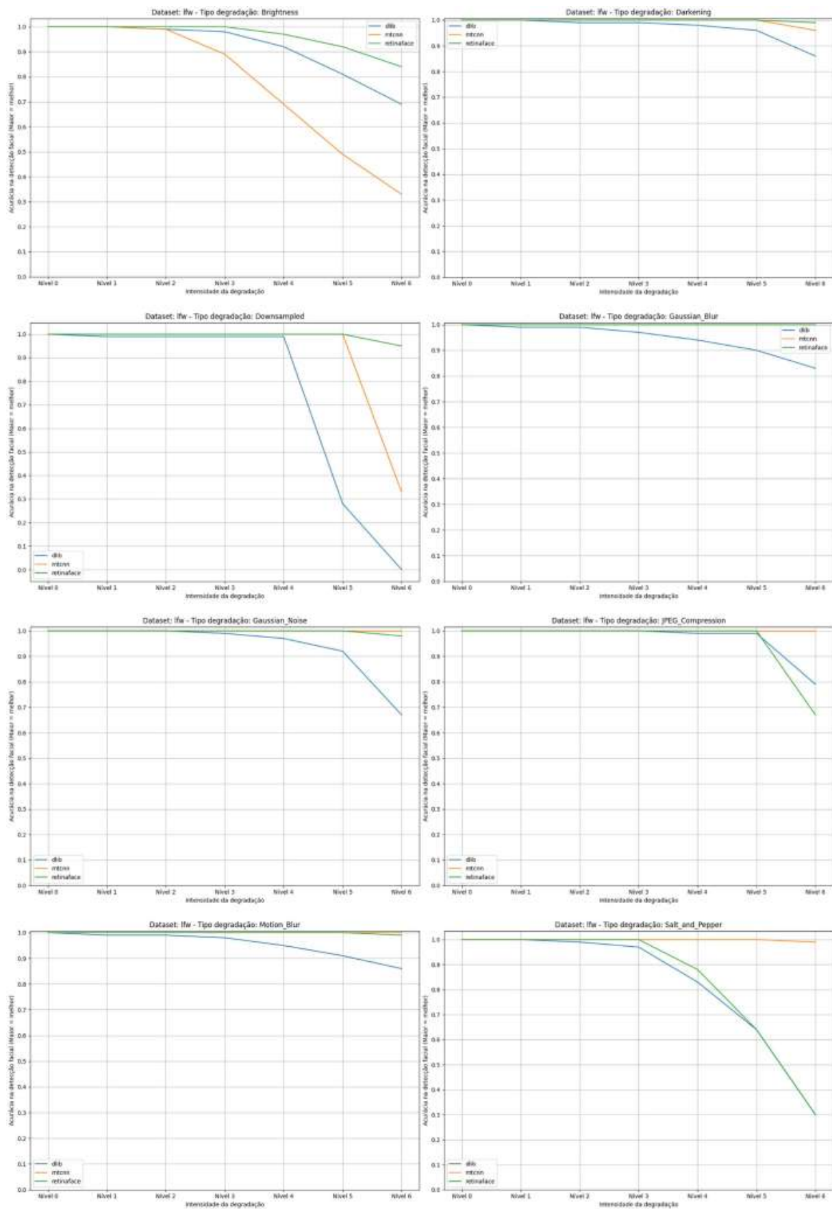
Figura 5.11: Desempenho dos algoritmos de detecção facial (degradações simples)
