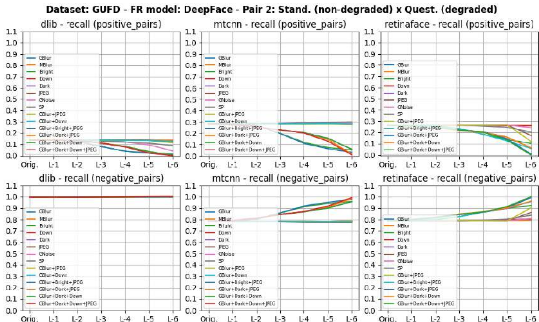
Figura I.58: Dataset GUFd - Par 2 - Métrica recall do algoritmo DeepFace
